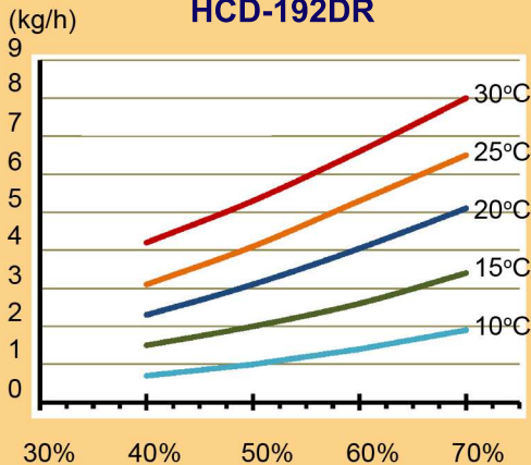
Biểu đồ công suất máy hút ẩm HCD-192DR
